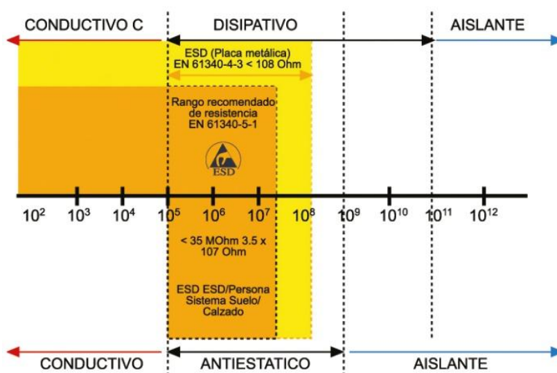
Sistema Suelo/Calzado usado como suelo para personal -Norma de ESD EN 61430
